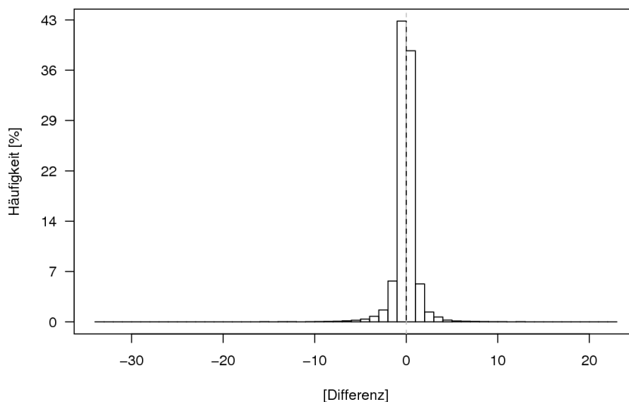
Abbildung 2.8: Häufigkeitsverteilung der Differenzen der stündlichen Niederschlagssummen von Beznau und Buchs/Aarau (Beznau minus Buchs/Aarau) in Klassen von 1 mm. Stunden, die an beiden Stationen keinen Niederschlag aufweisen, wurden für die Darstellung nicht verwendet.
