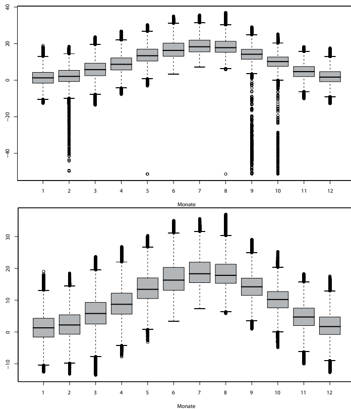
Abbildung 1.2: Temperatur Datenreihen von Beznau, 10 m Messniveau vor (oben) und nach (unten) der Datenbearbeitung.
