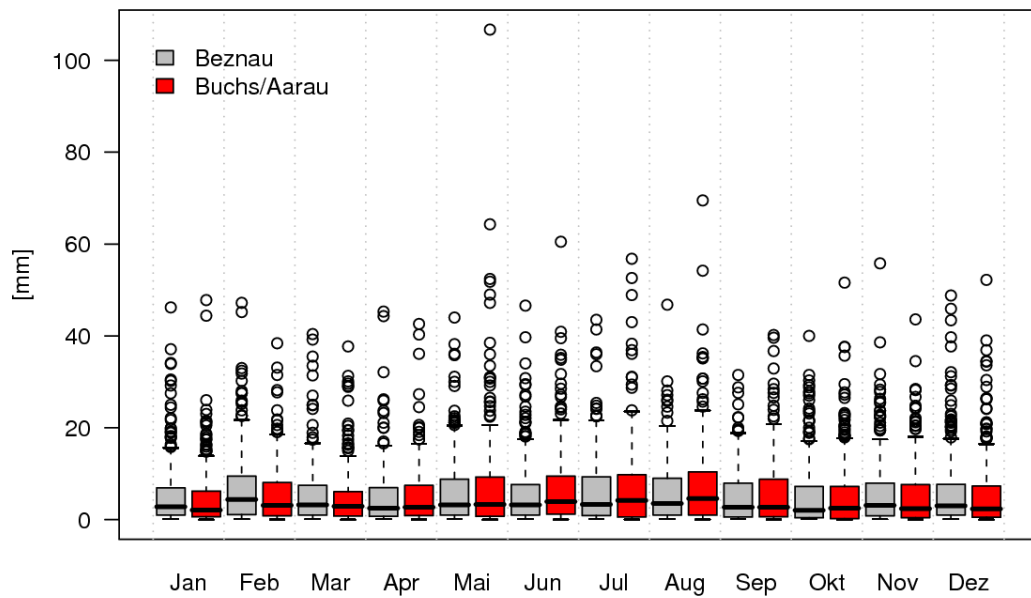
Abbildung 2.10: Gleich wie Abbildung 2.7 aber für die Tagessummen.
