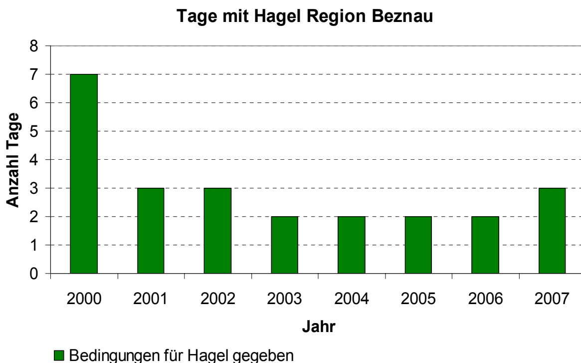
Abbildung 2.32: Anzahl Tage mit Hagel auf dem Gemeindegebiet des Standortes Beznau für die Jahre 2000 bis 2007.
