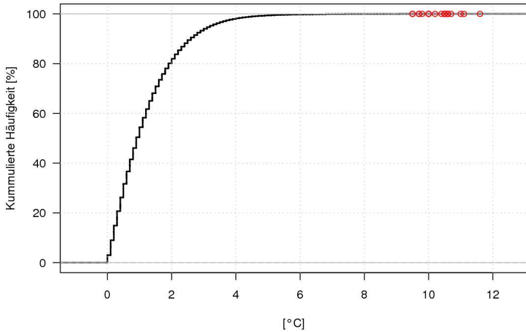
Abbildung 2.15: Kumulierte Häufigkeitsverteilung der absoluten Differenzen der Temperatur-Stundenmittel von Beznau und Basel/Binningen (Beznau minus Basel/Binningen). Es kann abgelesen werden, welcher Prozentsatz der Differenzen kleiner oder gleich einem bestimmten Wert ist. Die 20 grössten Differenzen sind mit roten Kreisen hervorgehoben.
