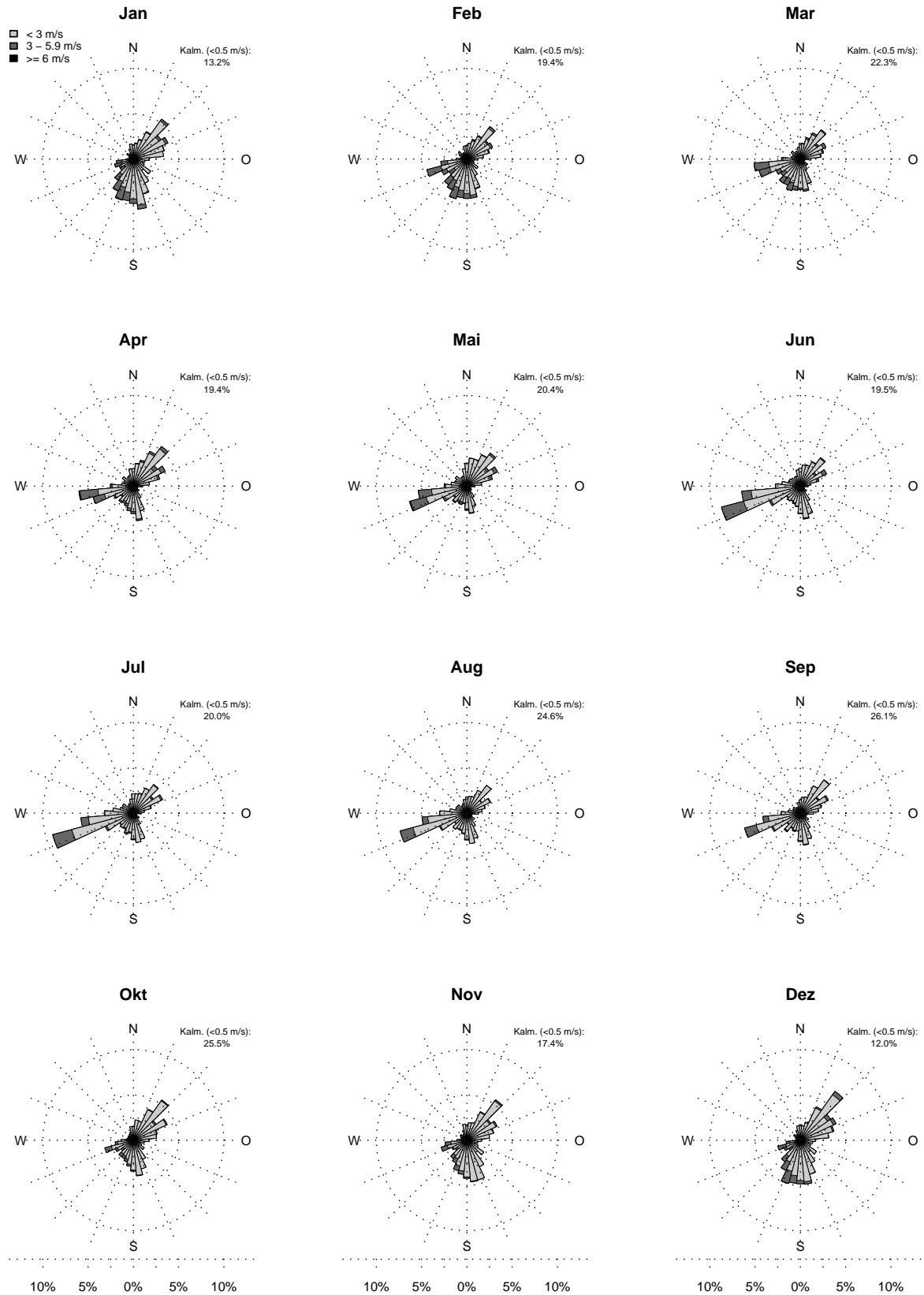
Abbildung 2.26: Mittlere monatliche Windrose der Periode 01.02.1987 bis 31.12.2007 am Standort Beznau auf dem Niveau 10 m über Grund auf Basis von Stundenmittelwerten. Die Grösse der Windrichtungsklassen beträgt 10 Grad. Windgeschwindigkeiten unter 0.5 m/s (Kalmen) werden nicht dargestellt.
