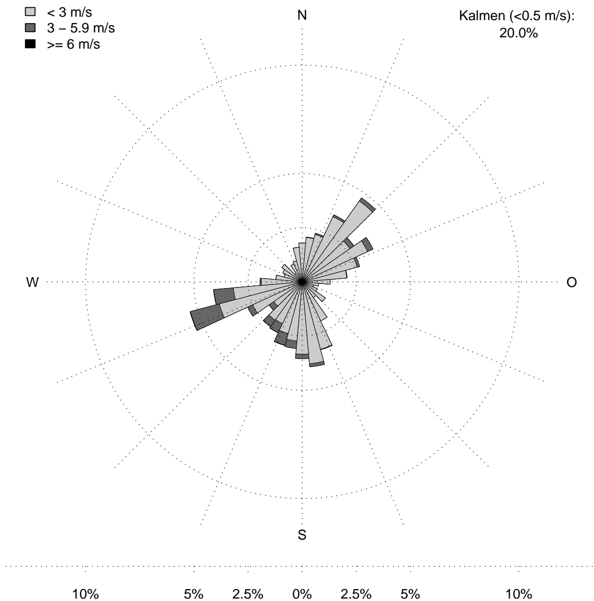
Abbildung 2.25: Mittlere jährliche Windrose der Periode 01.02.1987 bis 31.12.2007 am Standort Beznau auf dem Niveau 10 m über Grund auf Basis von Stundenmittelwerten. Die Grösse der Windrichtungsklassen beträgt 10 Grad. Windgeschwindigkeiten unter 0.5 m/s (Kalmen) werden nicht dargestellt.
