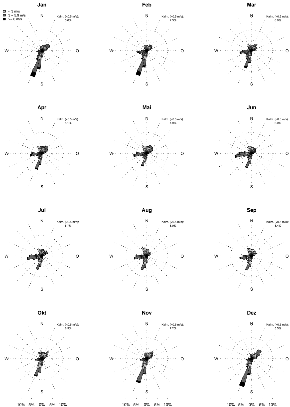
Abbildung 2.28: Mittlere monatliche Windrose der Periode 01.02.1987 bis 31.12.2007 am Standort Beznau auf dem Niveau 70 m über Grund auf Basis von Stundenmittelwerten. Die Grösse der Windrichtungsklassen beträgt 10 Grad. Windgeschwindigkeiten unter 0.5 m/s (Kalmen) werden nicht dargestellt.
