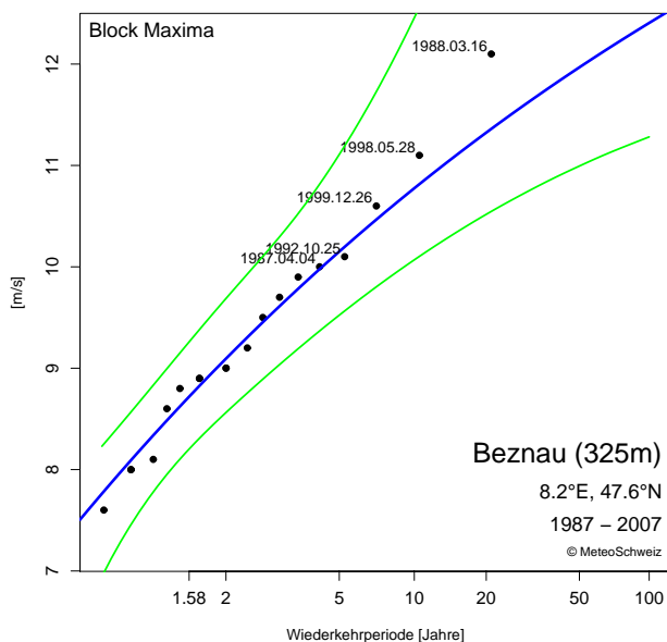
Abbildung 3.8: Gumbel-Diagramm an der Station Beznau für die 10-Minuten mittlere Windgeschwindigkeit auf dem 10 m Messniveau. GOF-Test: Da der GOF-Test nicht durchgeführt werden konnte, gibt es keine Angaben zur Güte des Fits. Grün: 90% Konfidenzintervall.
