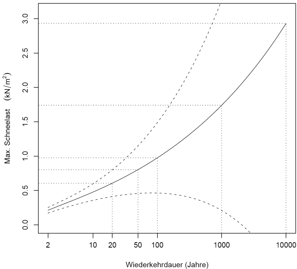
Abbildung 2.37: Extremwert-Diagramm für die Wiederkehrdauer von maximal auftretenden Schneelasten am Standort Beznau. Konfidenzintervalle sind nicht zuverlässig für Wiederkehrperioden die grösser sind als die zugrundeliegende Datenreihe selbst (vgl. Wiederkehrperiode > 100 Jahre). Eine Schneelast von ca. 0.81 \text{ kN/m}^2 hat an der Station Beznau eine Wiederkehrperiode von 50 Jahren. Zusätzlich zeigt die obere Grenze des 95% Konfidenzintervalls, das bei 95% der möglichen Verteilungen eine Schneelast von beispielsweise 0.81 \text{ kN/m}^2 eine Wiederkehrperiode von 20 Jahren haben kann.
