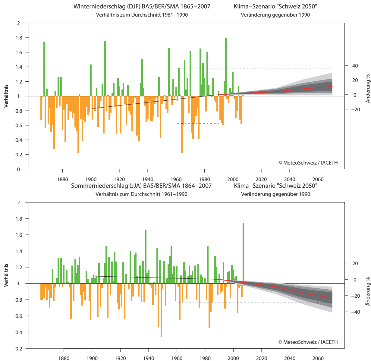
Abbildung 4.4: Wie Abbildung 4.3, aber für die Entwicklung der mittleren Niederschläge. Die Messungen sind als Verhältnis gegenüber der Norm 1961 bis 1990 (Skala links) angegeben, das Szenario als prozentuale Änderung gegenüber dem Mittel 1980 bis 1999 (Skala rechts)
