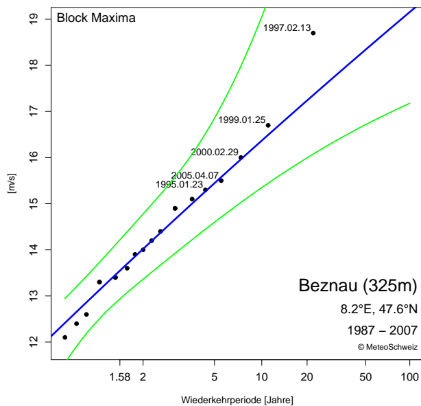
Abbildung 3.9: Gumbel-Diagramm an der Station Beznau für die 10-Minuten mittlere Windgeschwindigkeit auf dem 70 m Messniveau. GOF-Test: Da der GOF-Test nicht durchgeführt werden konnte, gibt es keine Angaben zur Güte des Fits. Grün: 90% Konfidenzintervall.
