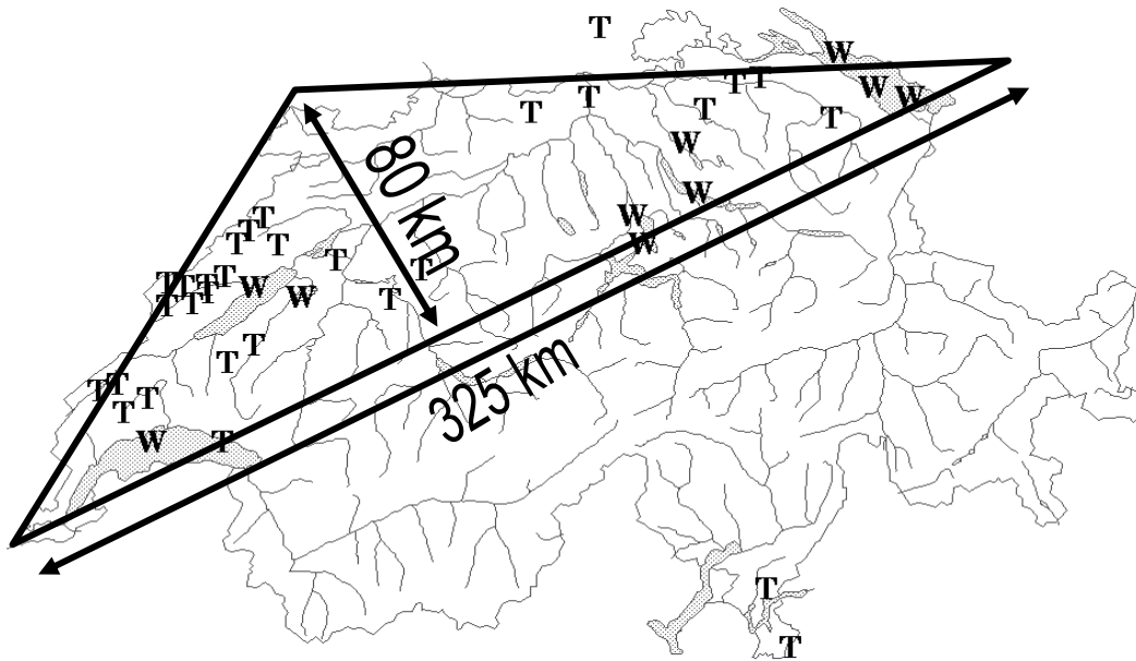
Abbildung 2.39: Die in der Nordschweiz von Tornados betroffene Region.
