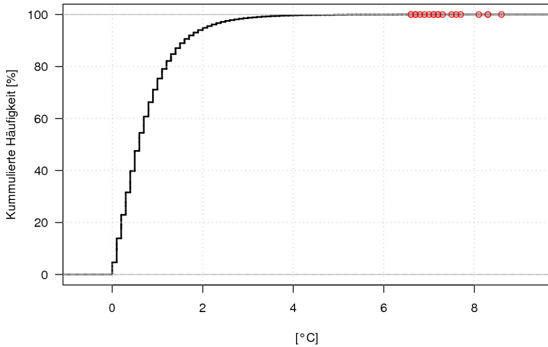
Abbildung 2.3: Kumulierte Häufigkeitsverteilung der absoluten Differenzen der Temperatur-Stundenmittel von Beznau und Buchs/Aarau (Beznau minus Buchs/Aarau). Es kann abgelesen werden, welcher Prozentsatz der Differenzen kleiner oder gleich einem bestimmten Wert ist. Die 20 grössten Differenzen sind mit roten Kreisen hervorgehoben.
