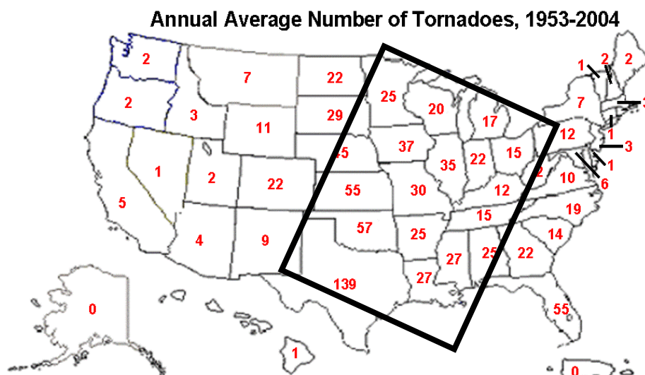
Abbildung 2.40: Jährliche Anzahl aller Tornados 1953 bis 2004 in den USA. Die schief liegende rechteckige Fläche (1500 km x 1800 km, 2.7 Mio. km 2 ) zeigt die Region mit der grössten Tornado-Dichte. Aus: http://wlf.ncdc.noaa.gov/oa/climate/severeweather/tornadoes.html
