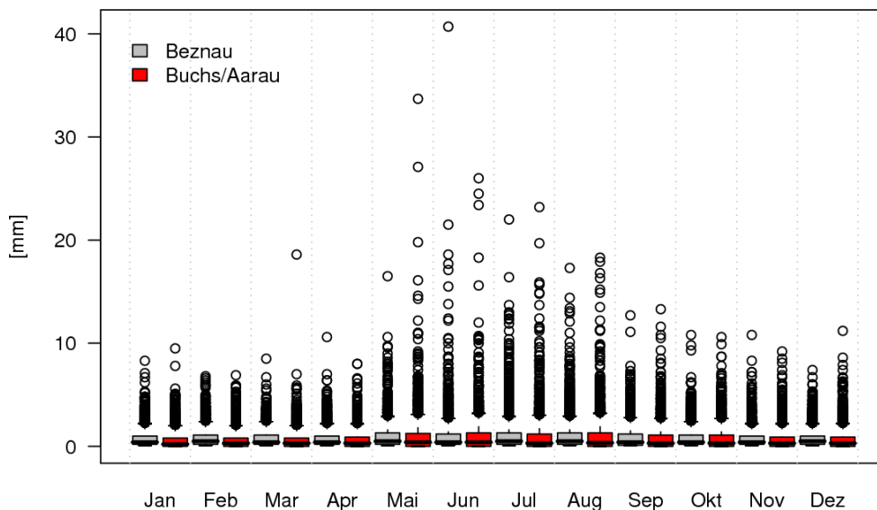
Abbildung 2.7: Vergleich der stündlichen Niederschlagssummen von Beznau und Buchs/Aarau in der Periode 12.10.1988 bis 31.12.2007. Die Boxplots zeigen die Verteilung der Stundenwerte separat an beiden Stationen für jeden Monat. Stunden ohne Niederschlag wurden für die Darstellung nicht berücksichtigt. Der Aufbau der Boxplots ist analog zu Abbildung 2.1. Da Niederschlagsmengen eine schiefe Verteilung aufweisen, ist die Vergleichbarkeit der Verteilungen mit Boxplots allerdings eingeschränkt.
