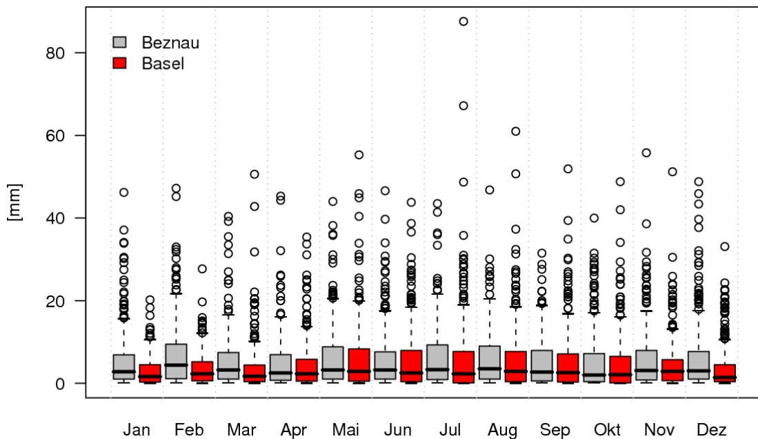
Abbildung 2.22: Gleich wie Abbildung 2.19 aber für die Tagessummen.
