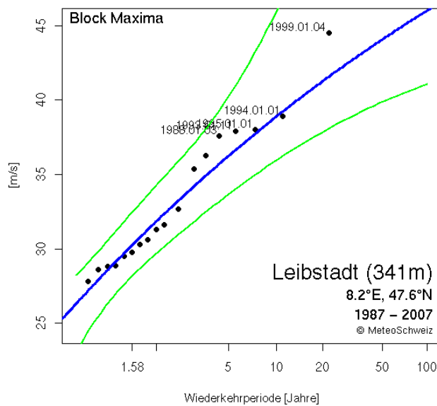
Abbildung 3.7: Gumbel-Diagramm an der Station Leibstadt für die 10-Minuten Böenspitze 110 m Messniveau. GOF-Test: Da der GOF-Test der Konfidenzintervalle nicht durchgeführt werden konnte, gibt es keine Angaben zur Güte des Fits. Grün: 90% Konfidenzintervall.
