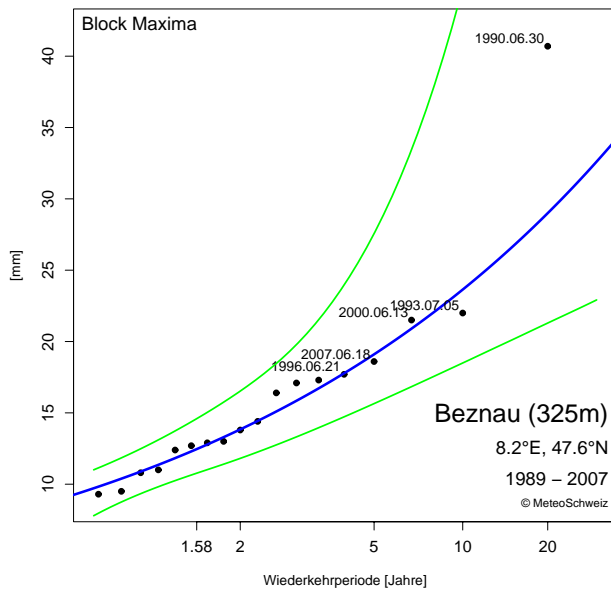
Abbildung 3.1: Gumbel-Diagramm an der Station Beznau für den stündlichen Niederschlag. GOF-Test: Die geschätzte Verteilung passt gut zu den Daten. Grün: 90% Konfidenzintervall.
