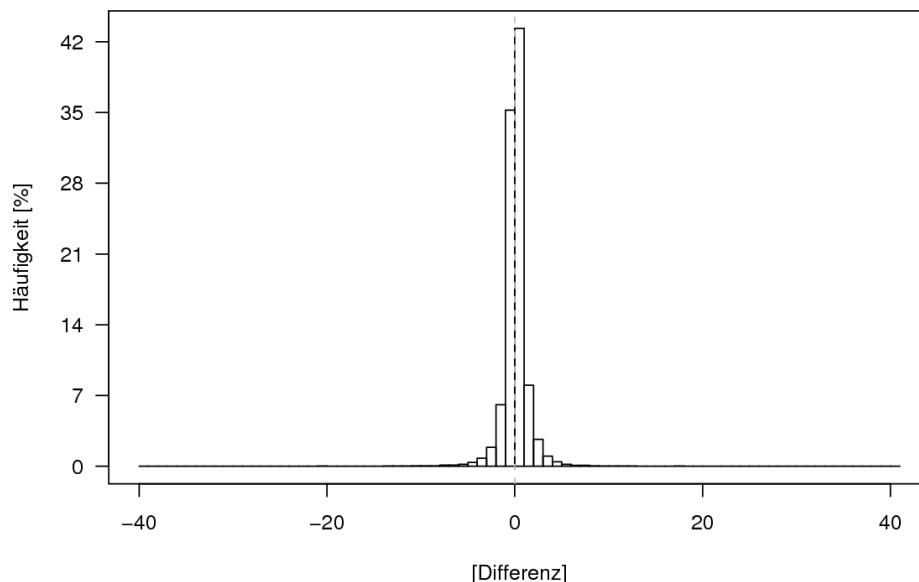
Abbildung 2.20: Häufigkeitsverteilung der Differenzen der stündlichen Niederschlagssummen von Beznau und Basel/Binningen (Beznau minus Basel/Binningen) in Klassen von 1 mm. Stunden, die an beiden Stationen keinen Niederschlag aufweisen, wurden für die Darstellung nicht verwendet.
