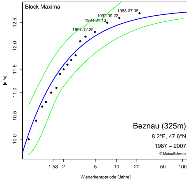
Abbildung 3.11: Gumbel-Diagramm an der Station Beznau für den Stundenmittel der Windgeschwindigkeit auf 70 m Messniveau. GOF-Test: da der GOF-Test nicht ausgeführt werden konnte, gibt es keine Angaben zur Güte vom Fit. Grün: 90% Konfidenzintervall.
