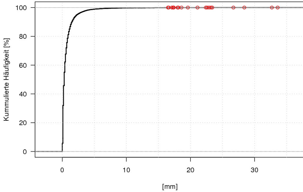
Abbildung 2.9: Kummulierte Häufigkeitsverteilung der absoluten Differenzen der stündlichen Niederschlagssummen von Beznau und Buchs/Aarau (Beznau minus Buchs/Aarau). Stunden, die an beiden Stationen keinen Niederschlag aufweisen, wurden für die Darstellung nicht verwendet. Es kann abgelesen werden, welcher Prozentsatz der Differenzen kleiner oder gleich einem bestimmten Wert ist. Die 20 grössten Differenzen sind mit roten Kreisen hervorgehoben.
