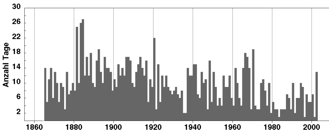
Abbildung 2.42: Anzahl Starkwindtage (Böenspitzen 90 km/h [50 Knoten] und mehr) im Winterhalbjahr für die Periode 1864/65 bis 2001/02 an der Messstation Zürich [49], (ergänzt). Die Station wird als repräsentativ für die Nordostschweiz angesehen. Einige umliegende Stationen wurden für Quervergleiche und für die Ergänzung fehlender Daten verwendet.
