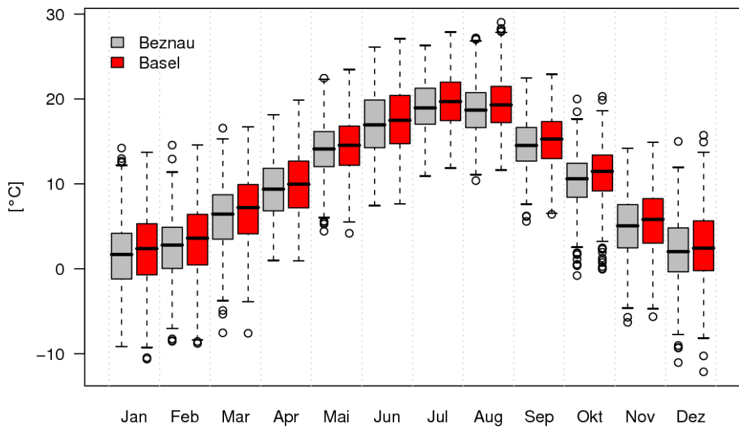
Abbildung 2.16: Gleich wie Abbildung 2.13 aber für die Tagesmittelwerte.
