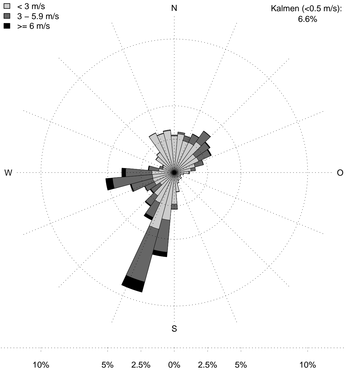
Abbildung 2.27: Mittlere jährliche Windrose der Periode 01.02.1987 bis 31.12.2007 am Standort Beznau auf dem Niveau 70 m über Grund auf Basis von Stundenmittelwerten. Die Grösse der Windrichtungsklassen beträgt 10 Grad. Windgeschwindigkeiten unter 0.5 m/s (Kalmen) werden nicht dargestellt.
