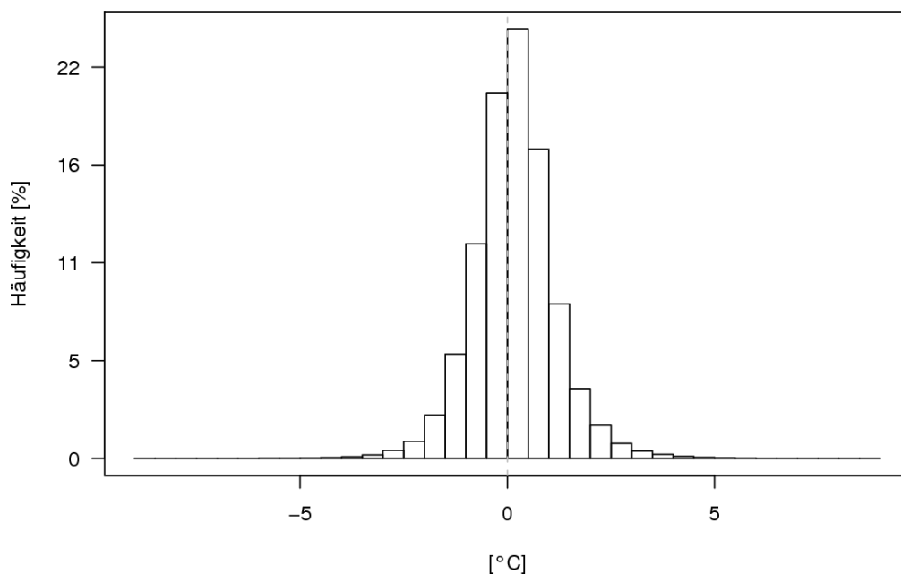
Abbildung 2.2: Häufigkeitsverteilung der Differenzen der Temperatur-Stundenmittel von Bezau und Buchs/Aarau (Bezau minus Buchs/Aarau) in Klassen von 0.5 Grad Celsius.
