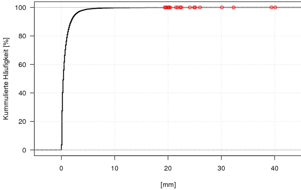
Abbildung 2.21: Kummulierte Häufigkeitsverteilung der absoluten Differenzen der stündlichen Niederschlagssummen von Beznau und Basel/Binningen (Beznau minus Basel/Binningen). Stunden, die an beiden Stationen keinen Niederschlag aufweisen, wurden für die Darstellung nicht verwendet. Es kann abgelesen werden, welcher Prozentsatz der Differenzen kleiner oder gleich einem bestimmten Wert ist. Die 20 grössten Differenzen sind mit roten Kreisen hervorgehoben.
