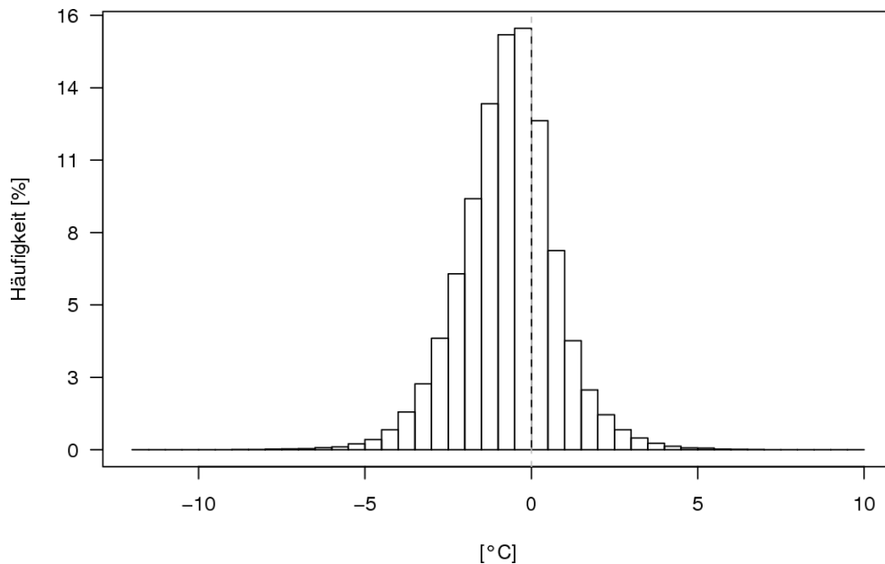
Abbildung 2.14: Häufigkeitsverteilung der Differenzen der Temperatur-Stundenmittel von Beznau und Basel/Binningen (Beznau minus Basel/Binningen) in Klassen von 0.5 Grad Celsius.
