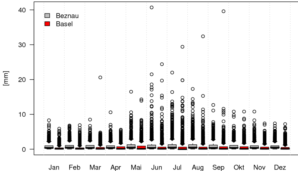
Abbildung 2.19: Vergleich der stündlichen Niederschlagssummen von Beznau und Basel/Binningen in der Periode vom 12.10.1988 bis 31.12.2007. Die Boxplots zeigen die Verteilung der Stundenwerte separat an beiden Stationen für jeden Monat. Stunden ohne Niederschlag wurden für die Darstellung nicht berücksichtigt. Der Aufbau der Boxplots ist analog zu Abbildung 2.13. Da Niederschlagsmengen eine schiefe Verteilung aufweisen, ist die Vergleichbarkeit der Verteilungen mit Boxplots allerdings eingeschränkt.
