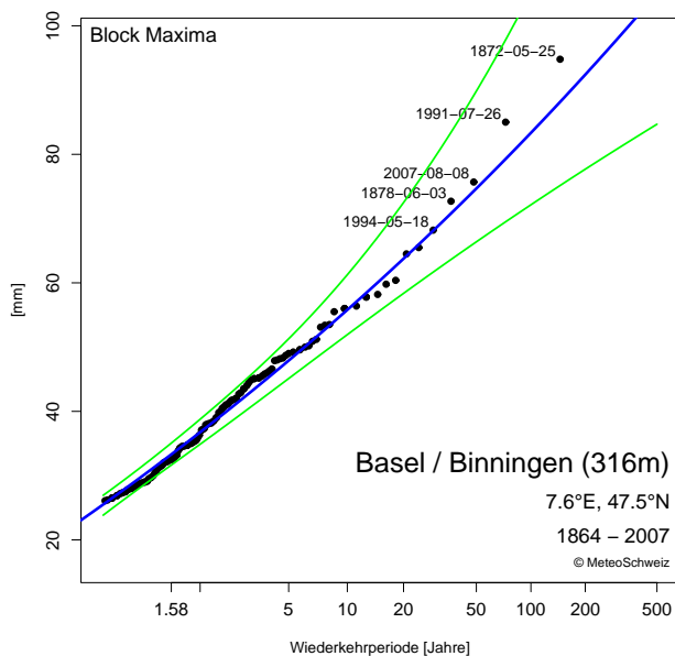
Abbildung 3.2: Gumbel-Diagramm an der Station Basel-Binningen 1-Tages Niederschlag. GOF-Test: Die geschätzte Verteilung passt gut zu den Daten. Grün: 90% Konfidenzintervall.
