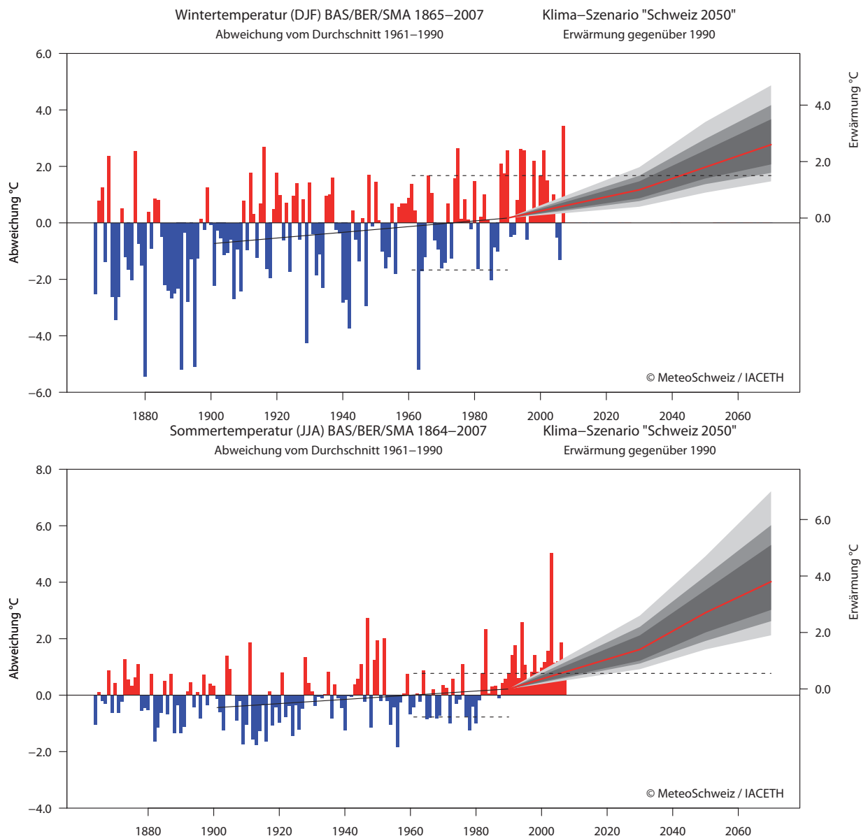
Abbildung 4.3: Entwicklung der mittleren Temperatur im Winter (Dezember bis Februar, oben) und im Sommer (Juni bis August, unten). Blaue/rote Säulen: gemessene Temperaturen für den Zeitraum 1864 bis 2007 (Mittel der Stationen Basel/Binningen, Bern/Zollikofen und Zürich/Fluntern, Abweichungen in Grad Celsius von der Norm 1961 bis 1990, Skala links). Schwarze Linie: linearer Trend 1901 bis 1990. Gestrichelte Linien: Bandbreite der Temperaturfluktuationen im heutigen Klima ( \pm 1 Standardabweichung) 1961 bis 1990. Graue Keile: erwartete zukünftige Änderung der mittleren Temperatur in der Nordschweiz bis 2070 (Änderung gegenüber dem Mittel 1980 bis 1999 in Grad Celsius, Skala rechts). Dunkelgraue Bereiche bezeichnen wahrscheinlichere, hellgraue weniger wahrscheinliche Entwicklungen für den Fall, dass keine raschen Massnahmen zur Einschränkung von Treibhausgasemissionen umgesetzt werden (95% Unsicherheitsbereich).
