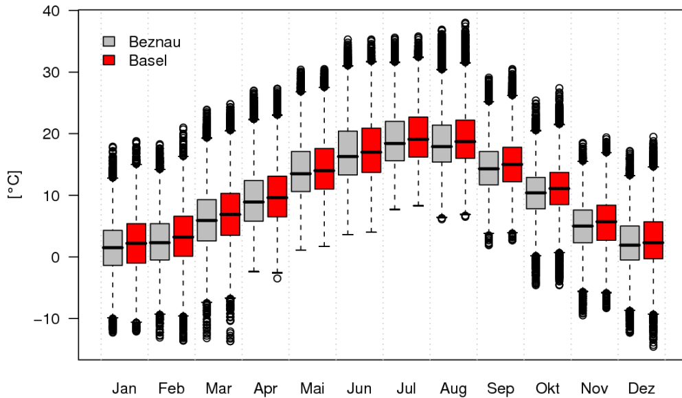
Abbildung 2.13: Vergleich der stündlichen Temperaturmittel von Beznau und Basel/Binningen in der Periode 1.2.1987 bis 31.12.2007. Die Boxplots zeigen die Verteilung der Stundenwerte separat an beiden Stationen für jeden Monat. Die Box der Boxplots umfasst die Messwerte zwischen dem 25%- und dem 75%-Quantil. Der Median wird durch eine Linie repräsentiert. Die sog. Whiskers (gestrichelte Linien) decken 1.5-mal die Box-Spannbreite gegen oben und unten ab und zeigen den Wertebereich der meisten Stundenwerte im entsprechenden Monat. Werte ausserhalb dieser Spannbreite können als Extremwerte bezeichnet werden und sind als Punkte einzeln dargestellt.
